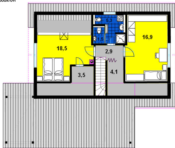
Půdorys podkrovní
